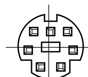
ミニ DIN-7J
