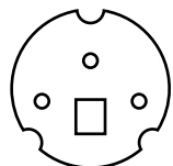
ミニ DIN-3P
